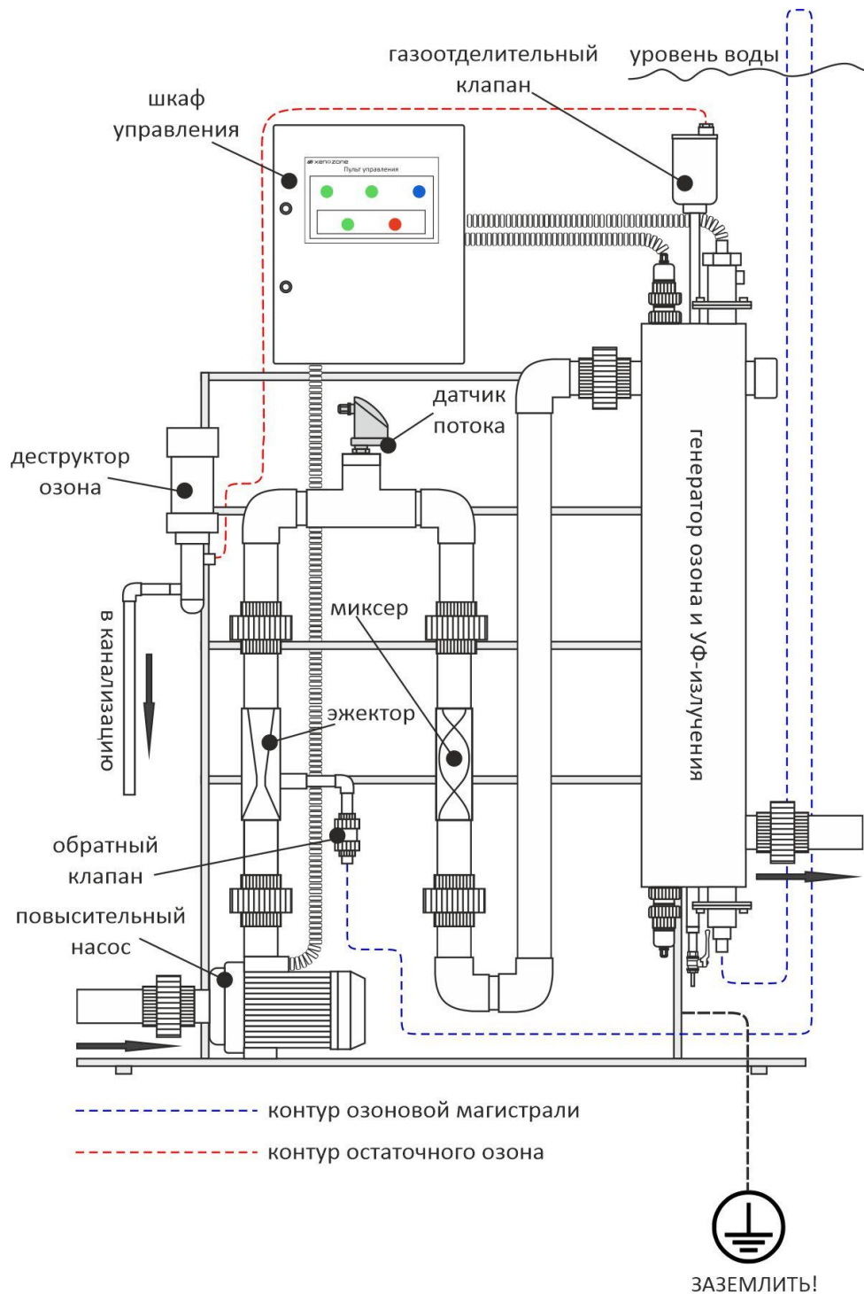
Схема компоновки устройств в составе системы
